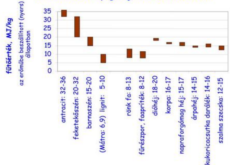
Szilárd tüzelőanyagok jellemző fűtőértékei
