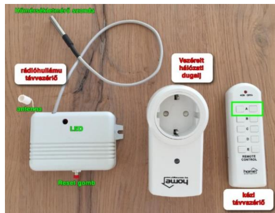
Tűztér hőmérséklet érzékelő – pl. kandalló és konyhai szagelszívó együttes üzemének tiltására
